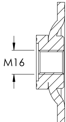
SCHNITT A-A
