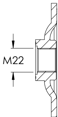
SCHNITT A-A
