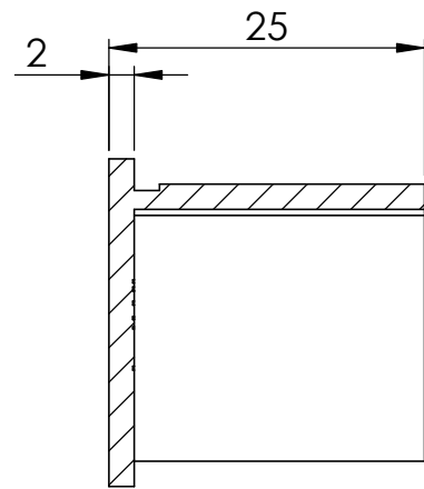
SCHNITT A-A
