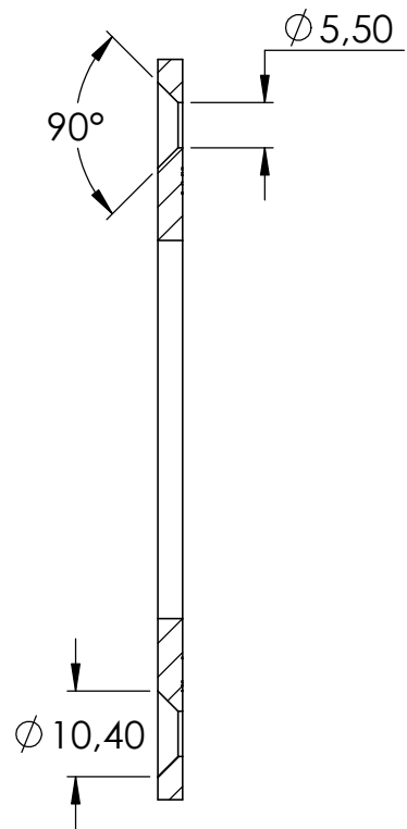
SCHNITT A-A
