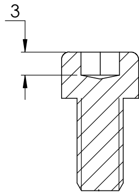
SCHNITT A-A
