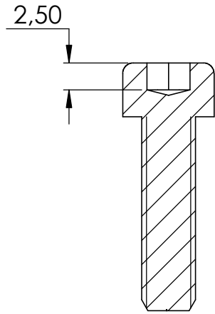
SCHNITT A-A
