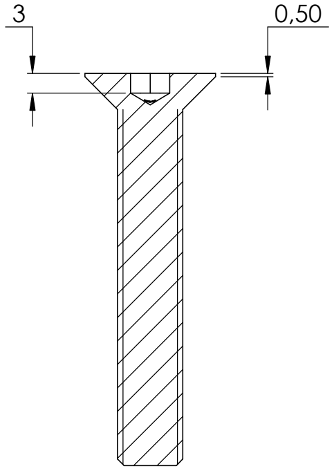
SCHNITT A-A
