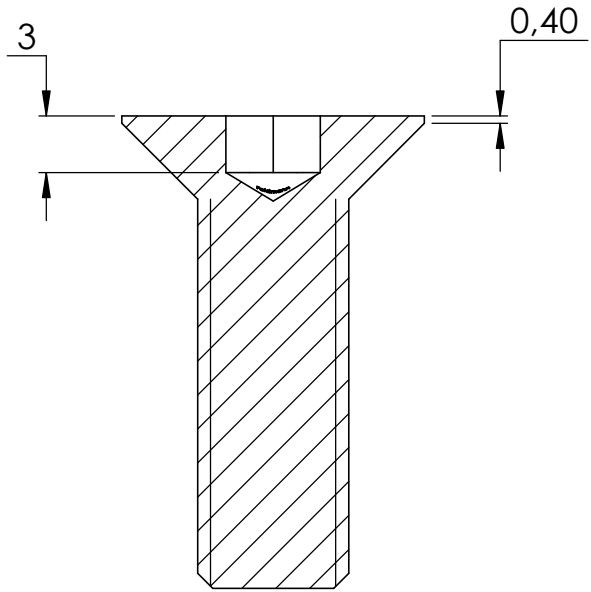
SCHNITT A-A
