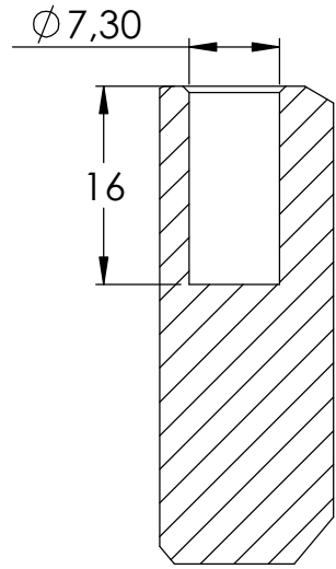
SCHNITT B-B
