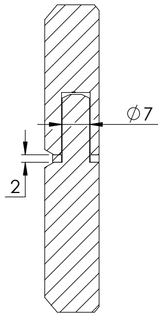
SCHNITT A-A
