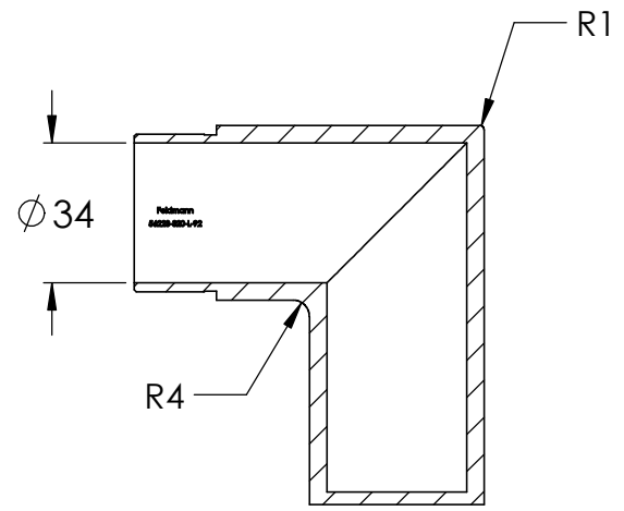
SCHNITT A-A
