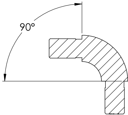
SCHNITT A-A
