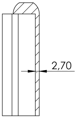
SCHNITT B-B
