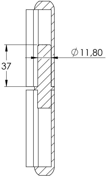
SCHNITT A-A
