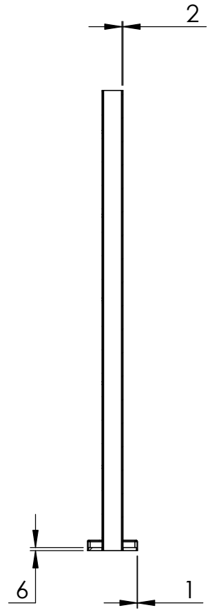
SCHNITT A-A
