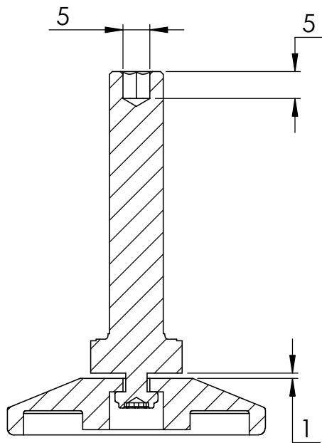
SCHNITT A-A
