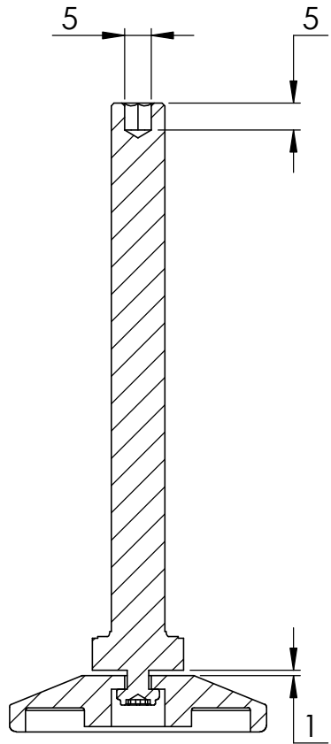
SCHNITT A-A
