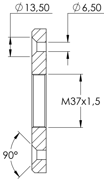
SCHNITT A-A
