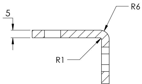
SCHNITT A-A
