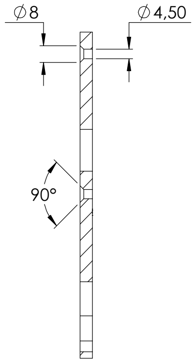
SCHNITT A-A
