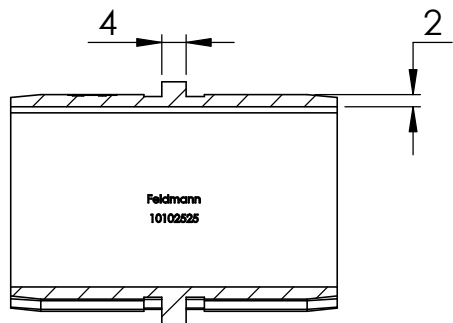
SCHNITT A-A
