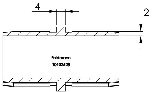
SCHNITT A-A
