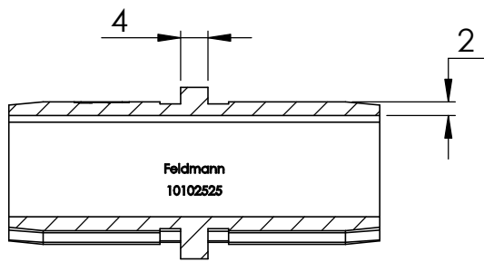
SCHNITT A-A
