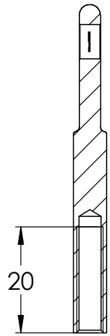
SCHNITT A-A
