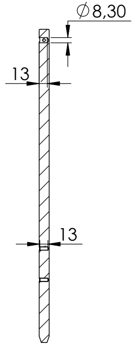
SCHNITT B-B
