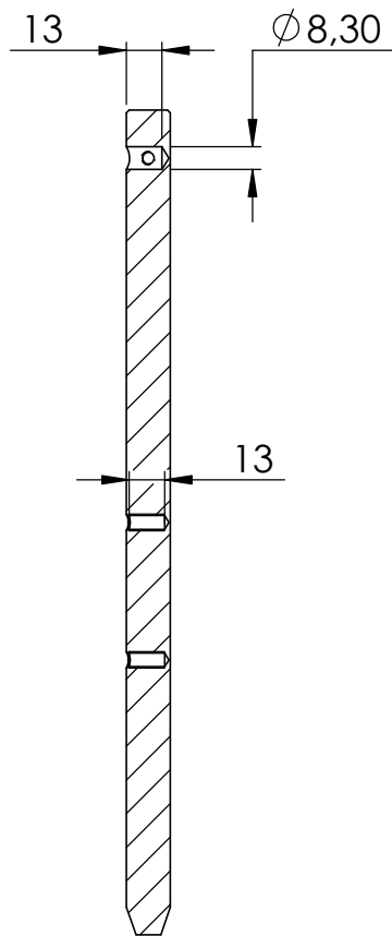
SCHNITT B-B
