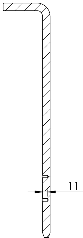
SCHNITT B-B
