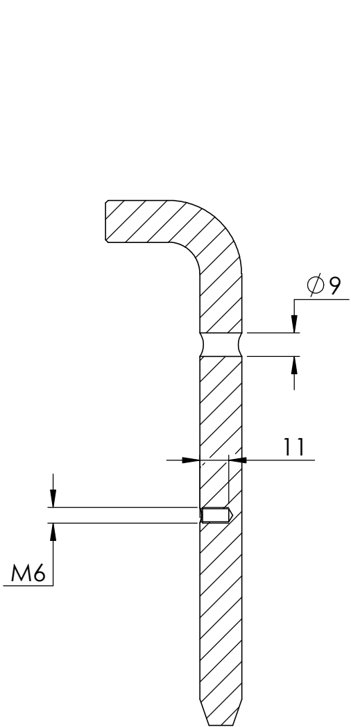
SCHNITT B-B
