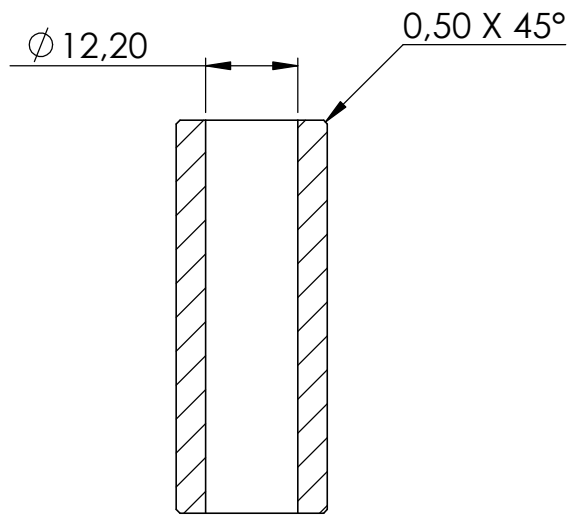
SCHNITT A-A
