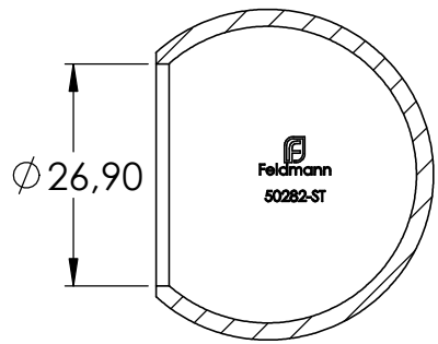
SCHNITT A-A
