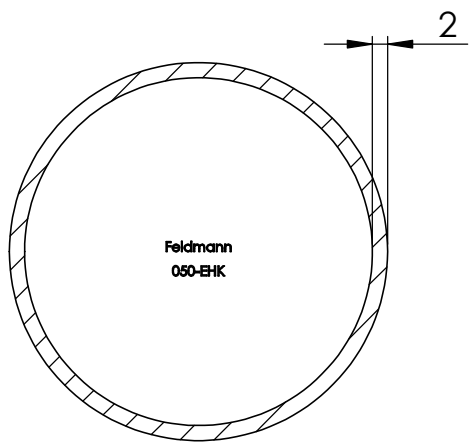
SCHNITT A-A
