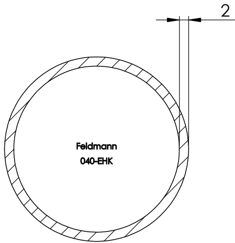
SCHNITT A-A
