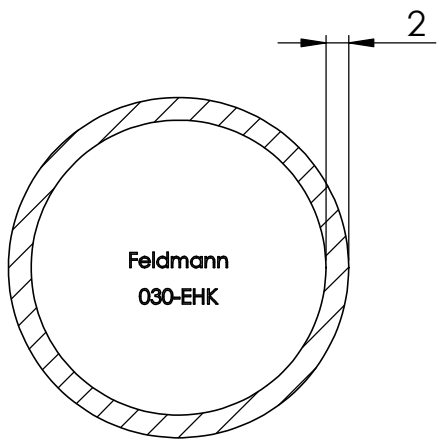
SCHNITT A-A
