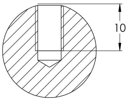
SCHNITT A-A
