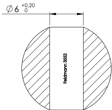
SCHNITT A-A
