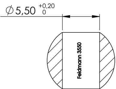
SCHNITT A-A
