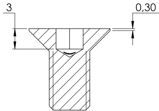
SCHNITT A-A
