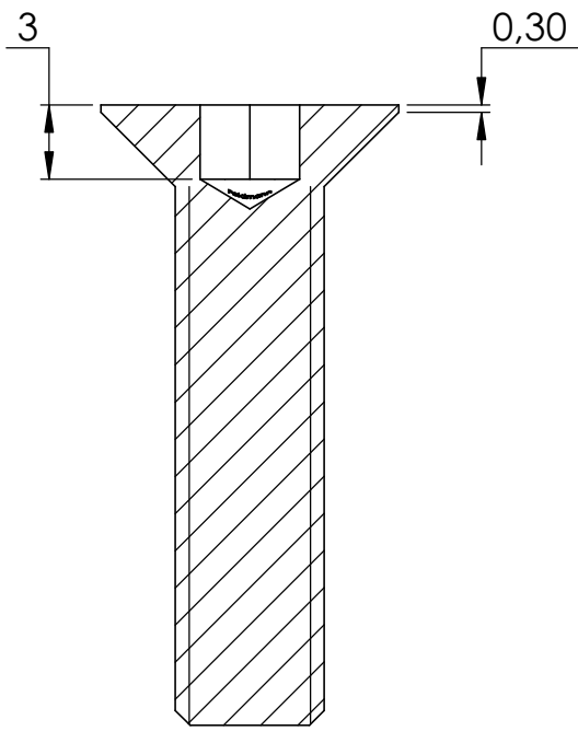
SCHNITT A-A
