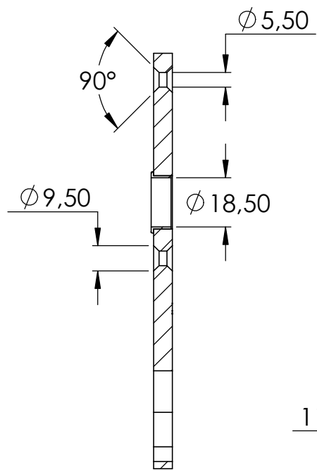
SCHNITT A-A
