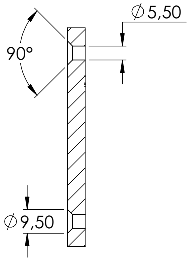
SCHNITT A-A
