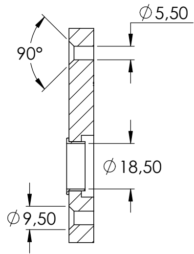
SCHNITT A-A
