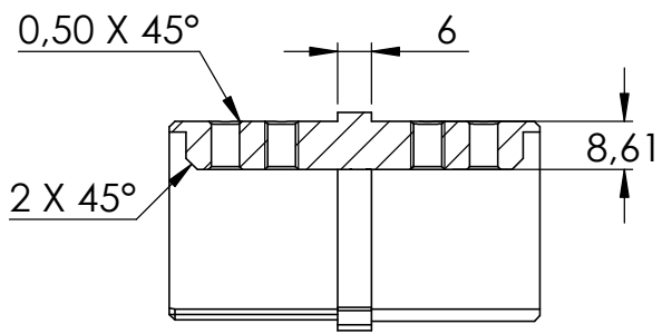
SCHNITT A-A
