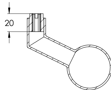
SCHNITT B-B
