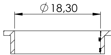
SCHNITT A-A
