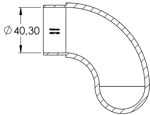
SCHNITT A-A
