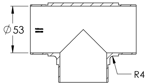
SCHNITT A-A
