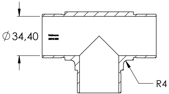
SCHNITT A-A
