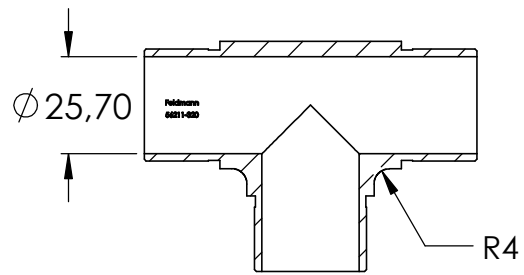
SCHNITT A-A
