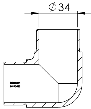
SCHNITT A-A
