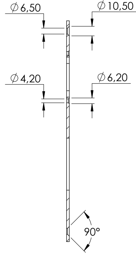
SCHNITT A-A
