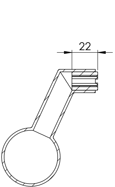
SCHNITT A-A
