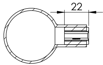
SCHNITT A-A
